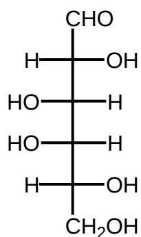
D-Galactose
