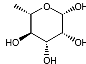
L-Rhamnose
