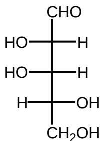
D-Lyxose
