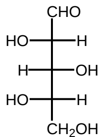
L-Arabinose
